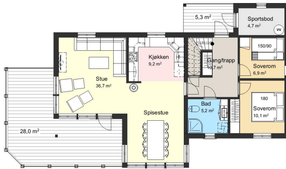
1:100 1. Etasje
