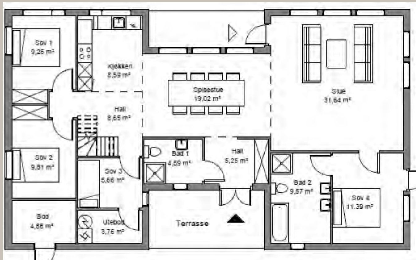
Hovedplan
