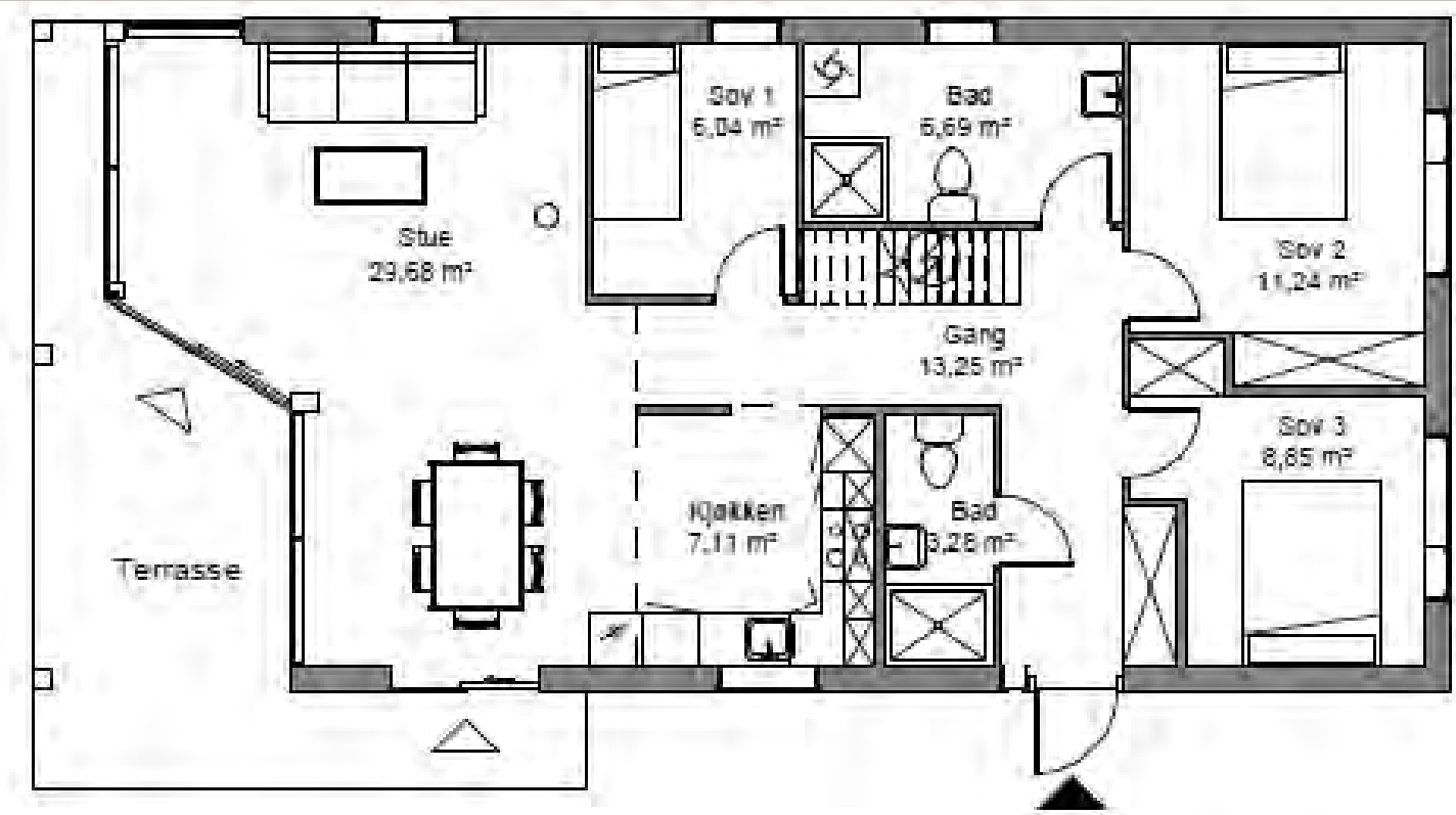
Hovedplan
