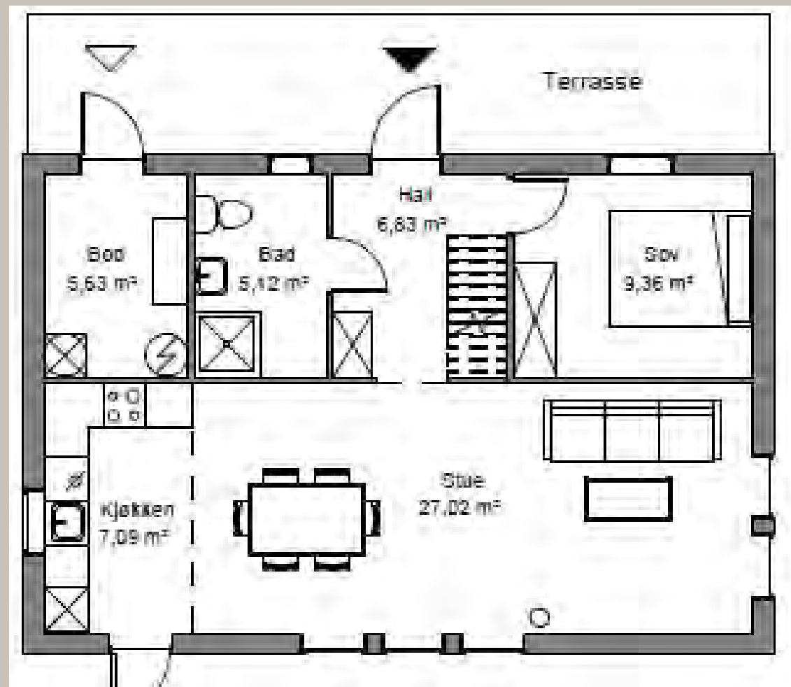
Hovedplan
