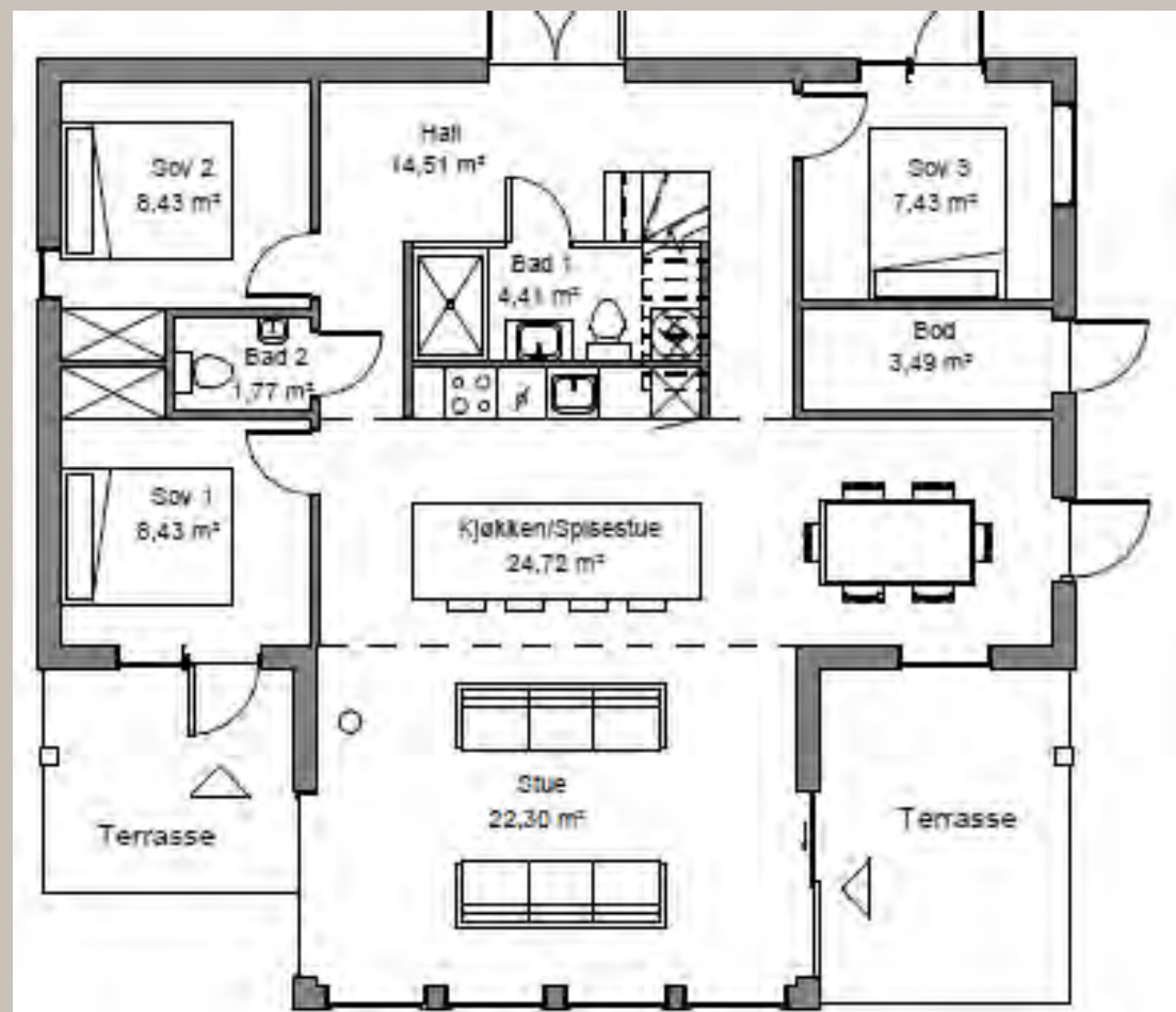
Hovedplan
